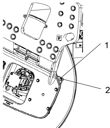
图：钢轮，振动侧视图 1. 橡胶件 2. 止动螺钉
