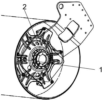
图例：油位检查 - 钢轮齿轮 1. 油位塞 2. 过滤器塞
