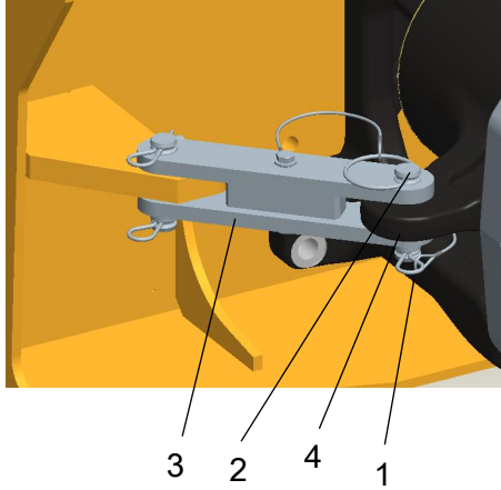
图：处于锁定位置的联结关节
