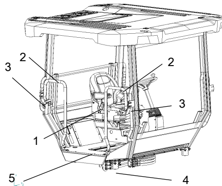
图：操作人员位置 1. 安全带 2. 防护栏 3. 锁扭 4. 橡胶件 5. 防滑保护装置
