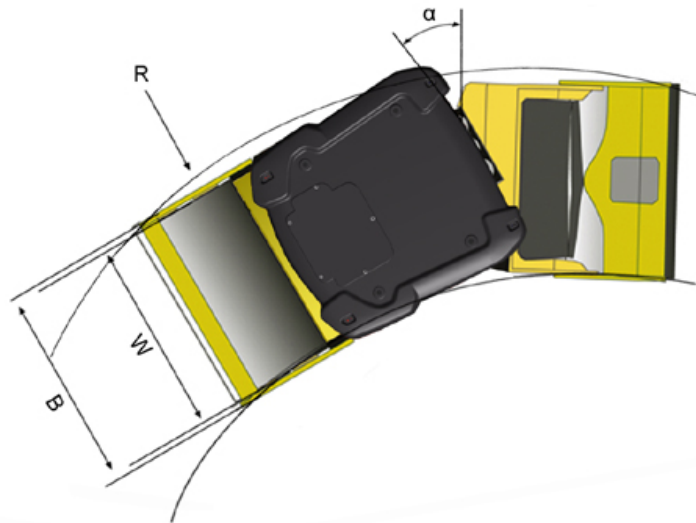
尺寸，俯视图
