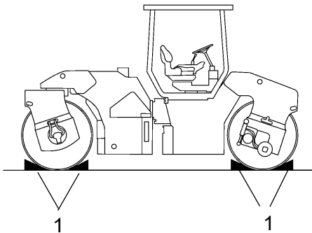
图 定位 1. 塞块
