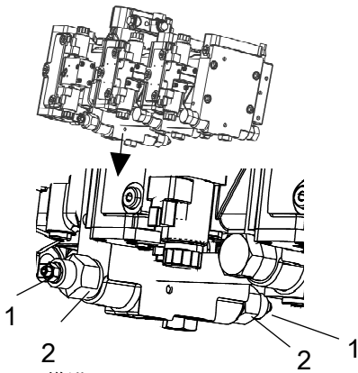
图：推进泵 1. 牵引阀 2. 旁通阀
